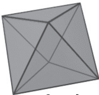
Октаедър
