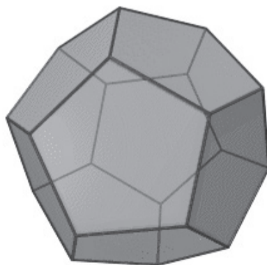
Додекаедър
