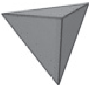
Тетраедър
