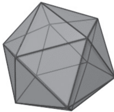
Икосаедър
